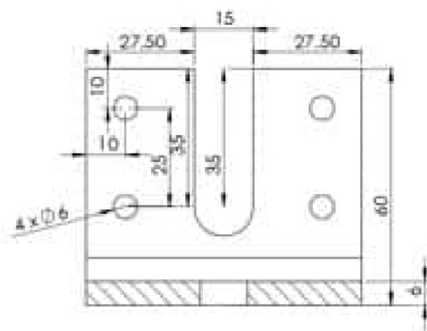
SEZIONE A-A
